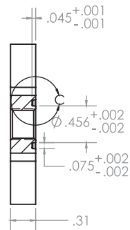
SECTION A-A
